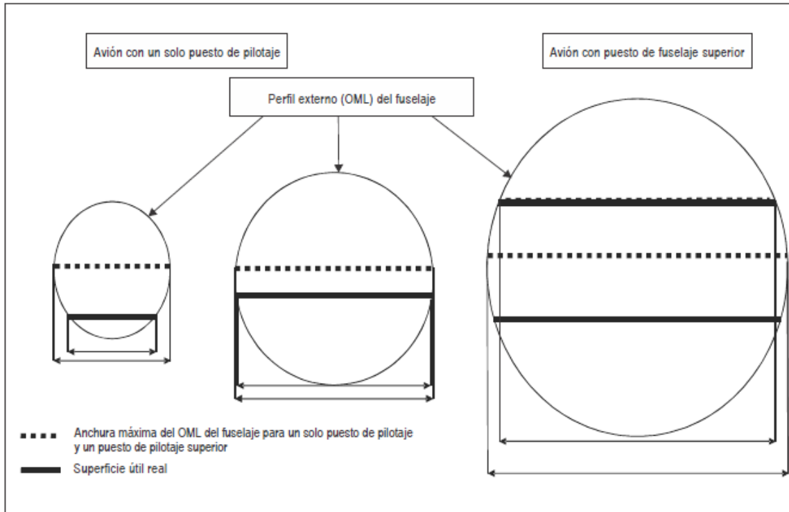
Figura A2-1 Vista Sección Transversal
