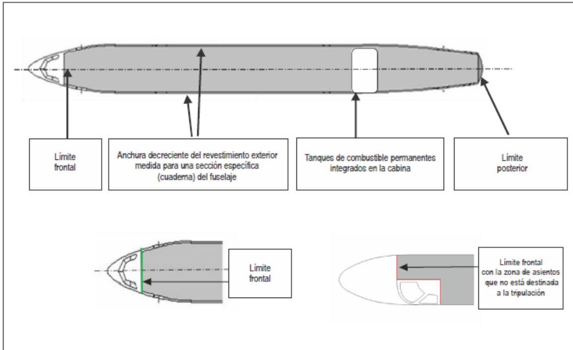
Figura A2-2 Vista en Planta
